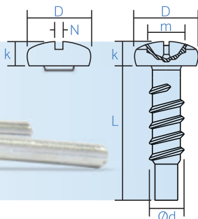
FENDA SIMPLES - DIN 7971
